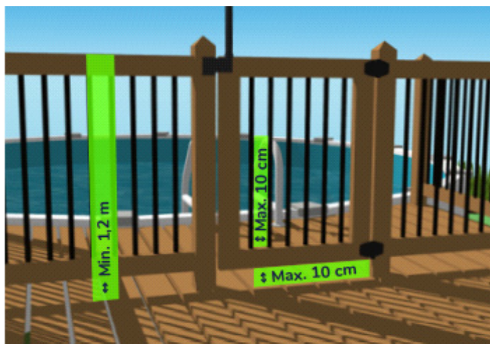
Dimensions exigées pour une enceinte.
